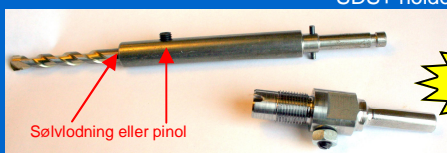
Forstærket 13 mm holder med lyn-kobling: 1JAPH005
